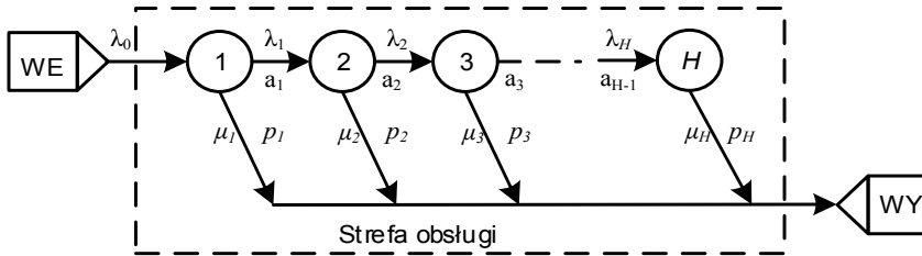
Rys. 8. SMO ze strefą obsługi (opracowanie własne na podstawie [6])
