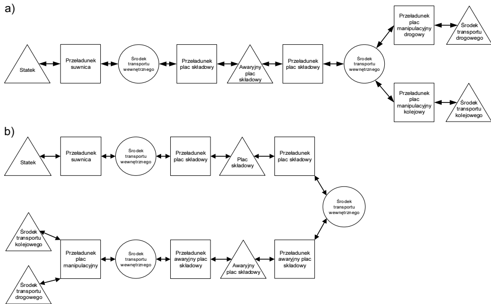
Rys. 6. Model obsługi awaryjnej CTU: a) w trakcie transportu wewnątrz terminalu, b) podczas składowania na placu składowym terminalu [7]
